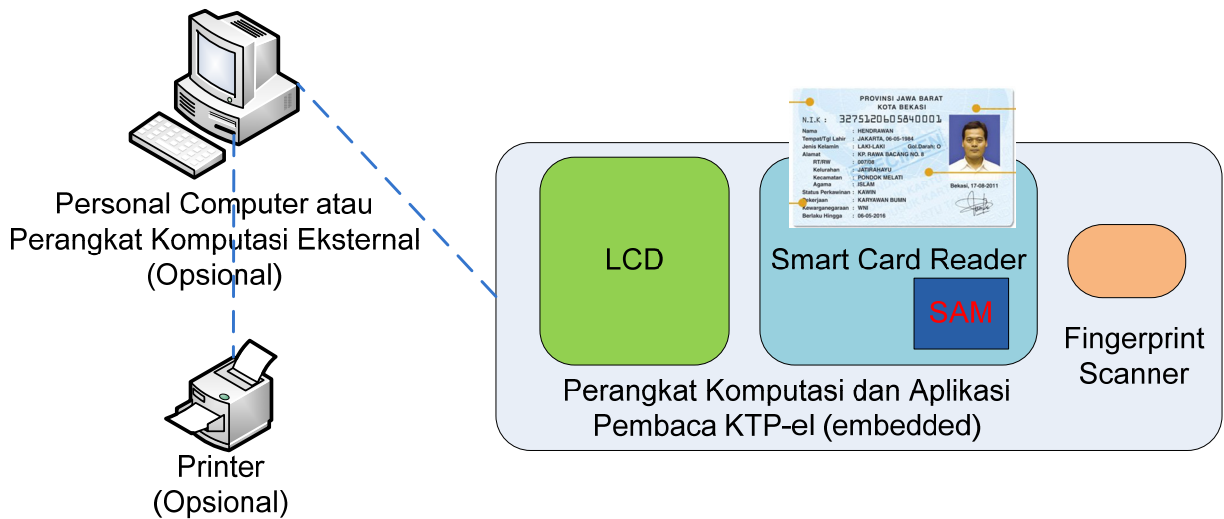
Gambar 2. Perangkat Pembaca KTP Elektronik Terintegrasi
